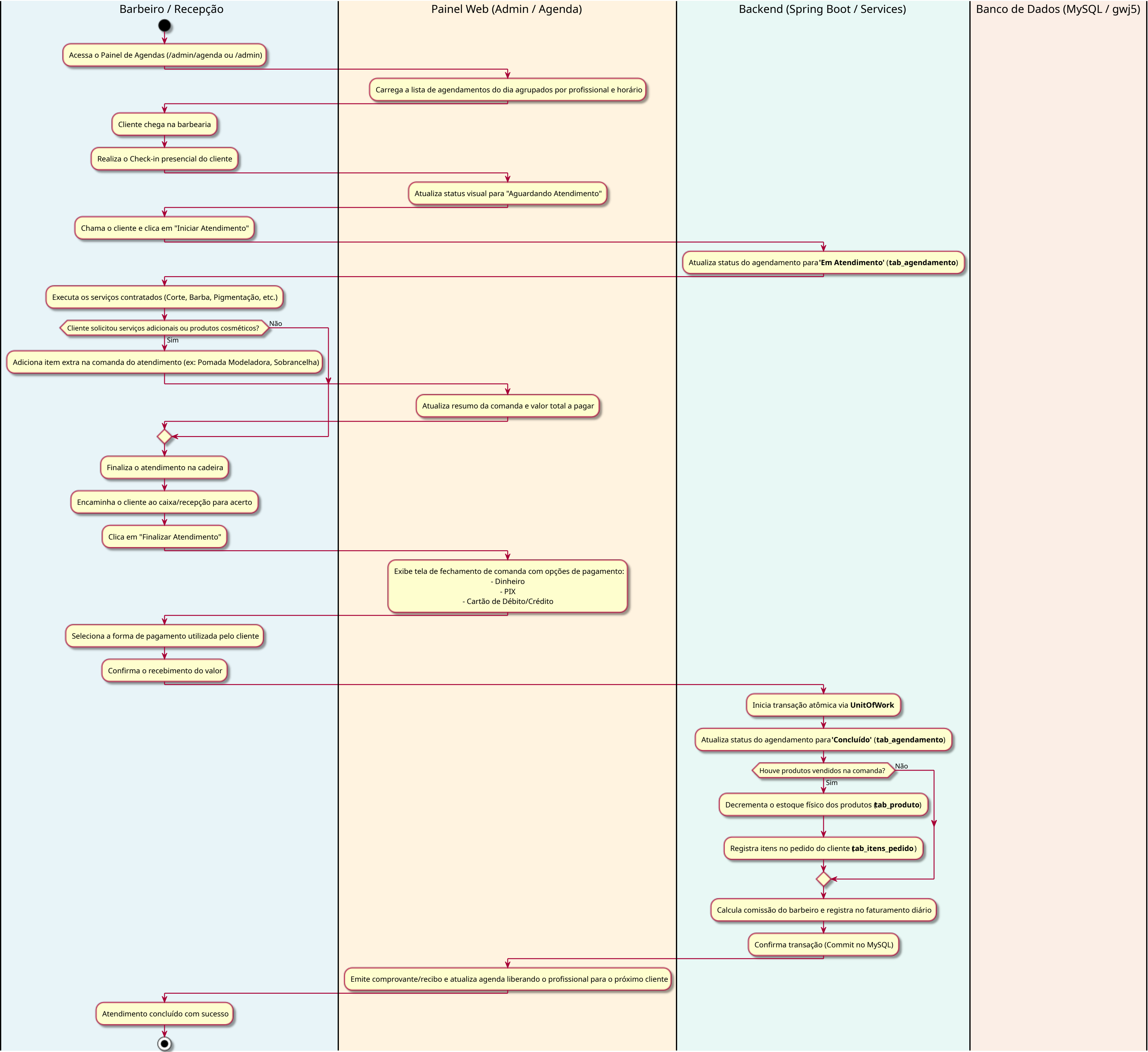
Diagrama de Atividades - Atendimento Presencial, Execução e Conclusão do Serviço
